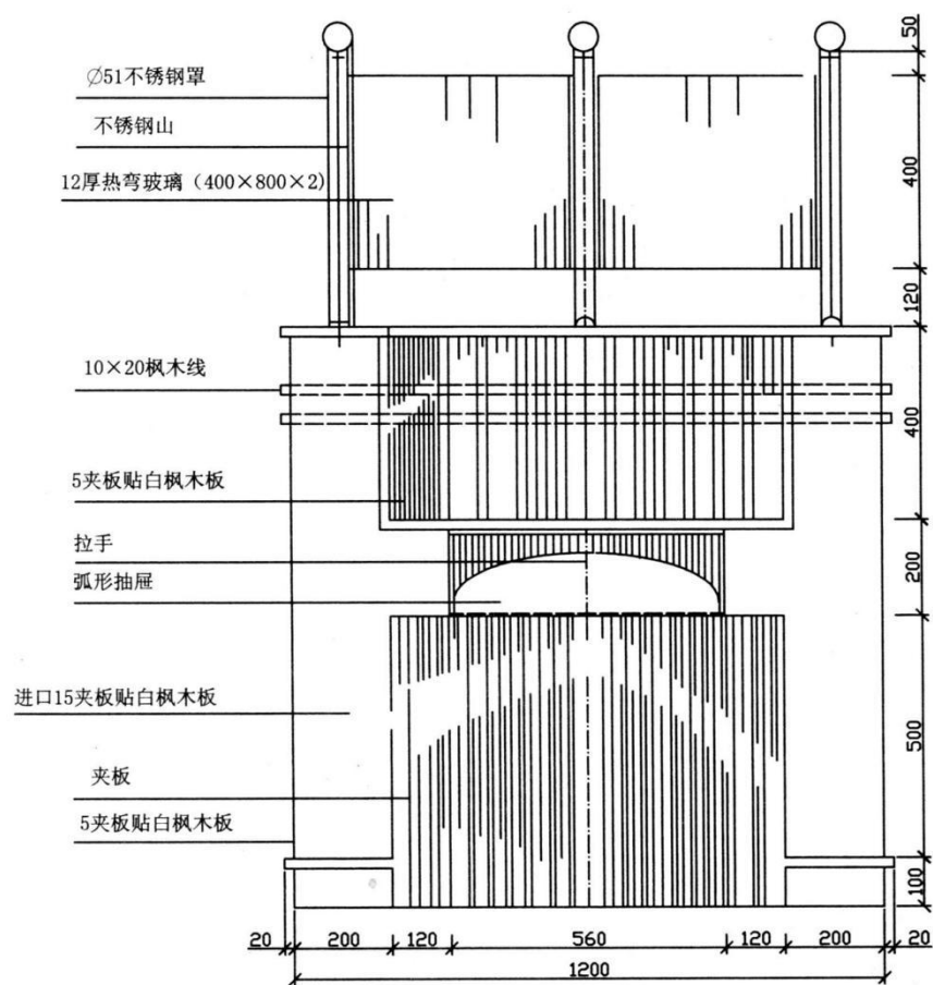
收银台立面
