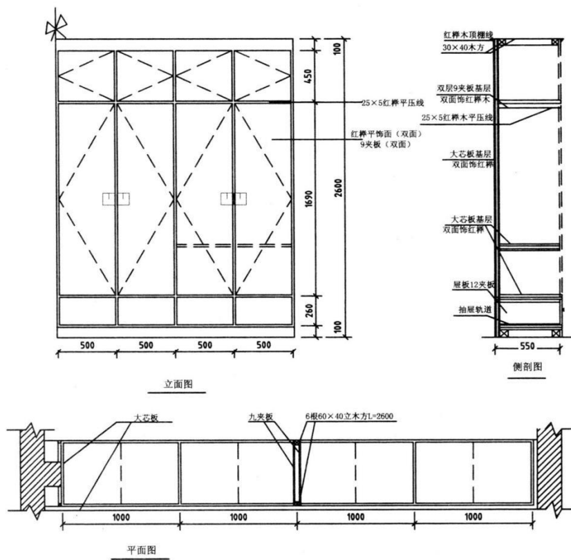
16-103 隔断木衣柜
