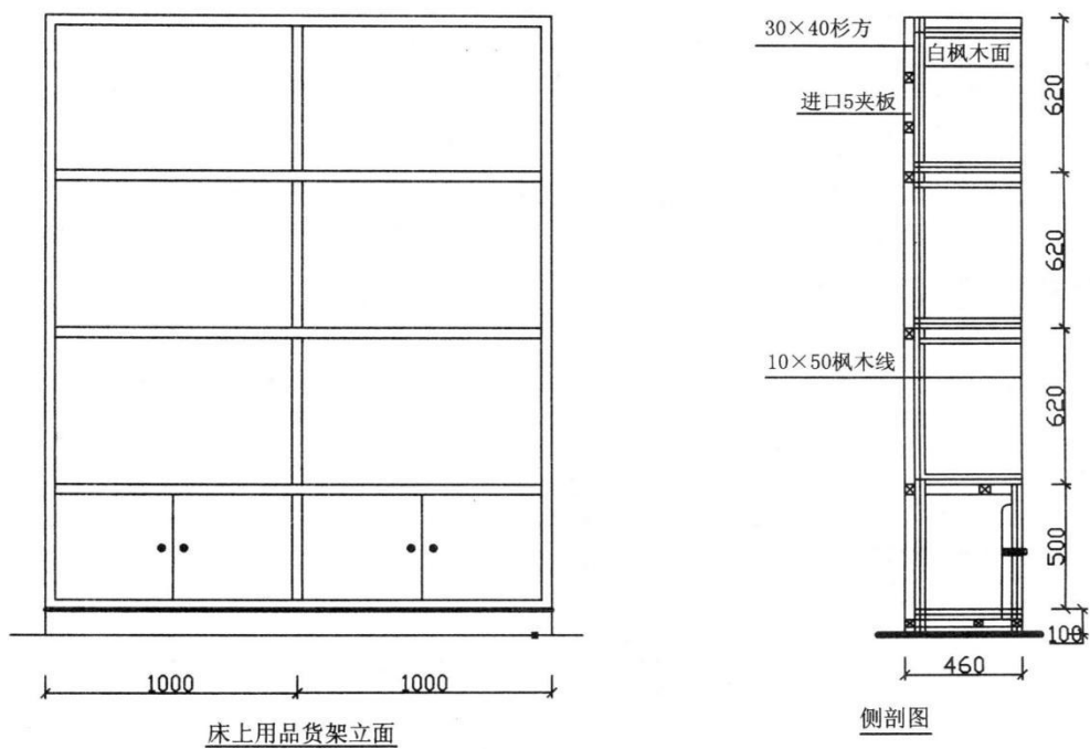
16-90 货架2
