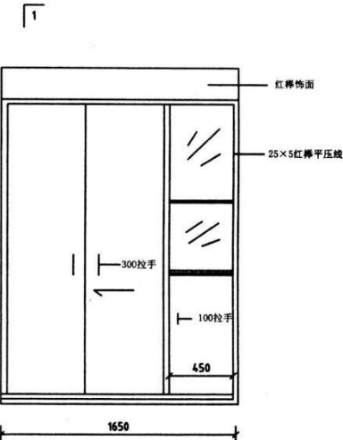
酒柜立面图
